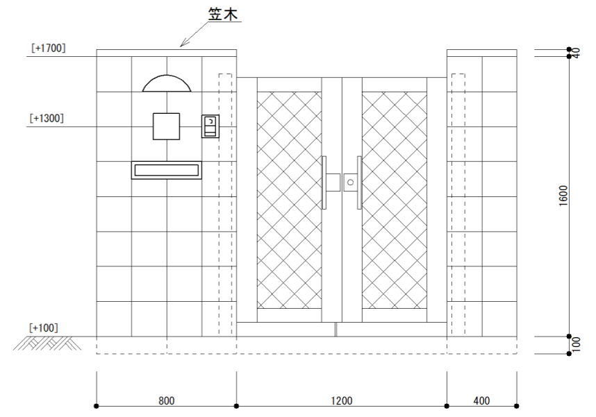
門扉詳細図 S=1/30
