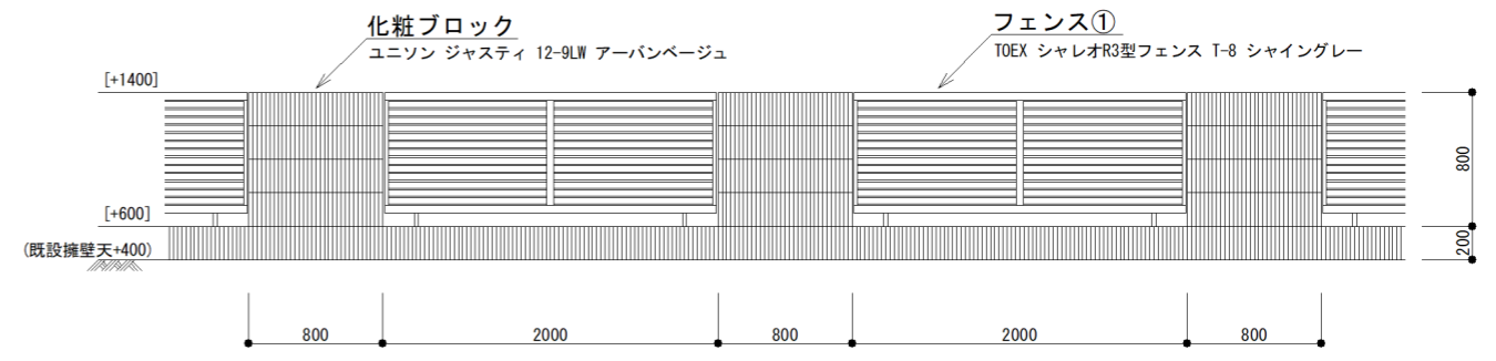
立面図 S=1/50
