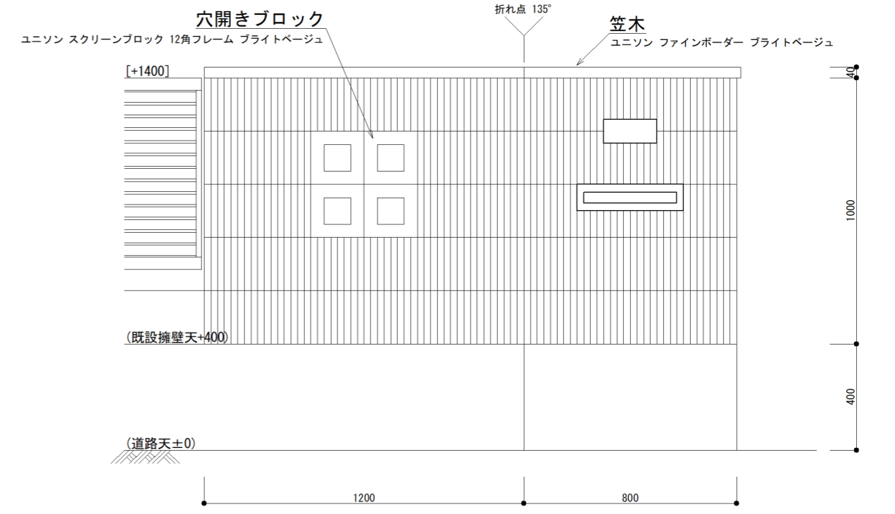
門扉正面図 S=1/20
